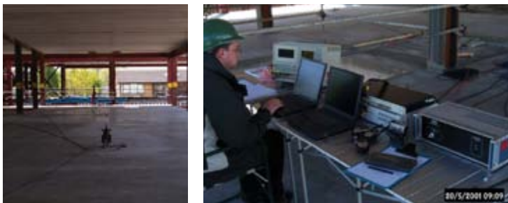
Динамичко испитивање међуспратне конструкције
