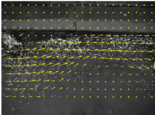
Slika 11: Konačno strujno polje (uklonjen šum slike)
